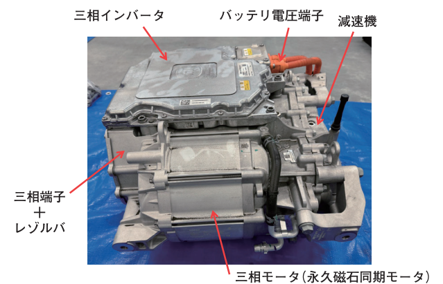
図3 SU7用 e-Axle
